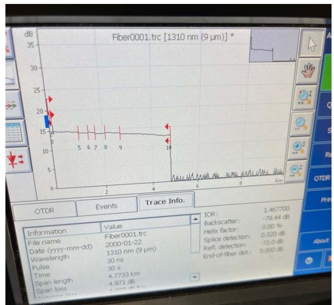
Figure 2 - Confirmation d'une coupure pour le lien de redondance à 4.7 km
