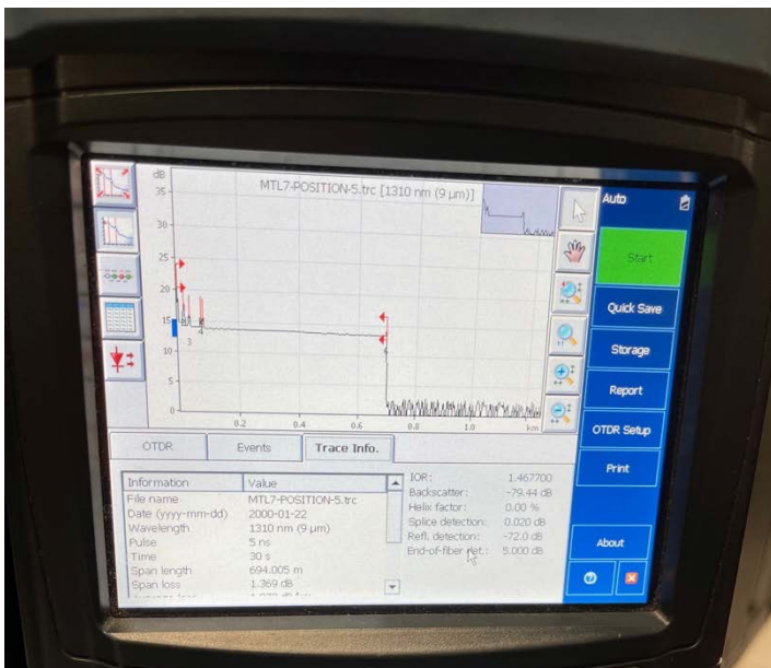
Figure 1 - Confirmation d'une coupure du lien principal à 694m
